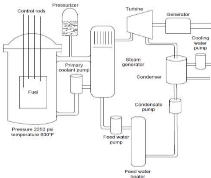
(۱- شکل): د هستوي ریاکتور اساسي برخې را په گوته کوي [۷: ۱۶۸].
