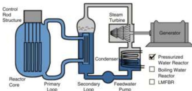
(۳-شکل): د فشار لاندې سپکو اوبو ریاکتور یوه وصفي منظره [۱۲].
